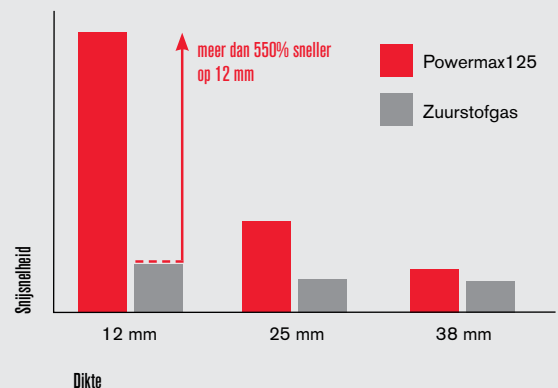
Relatieve snijprestatie op koolstofstaal
